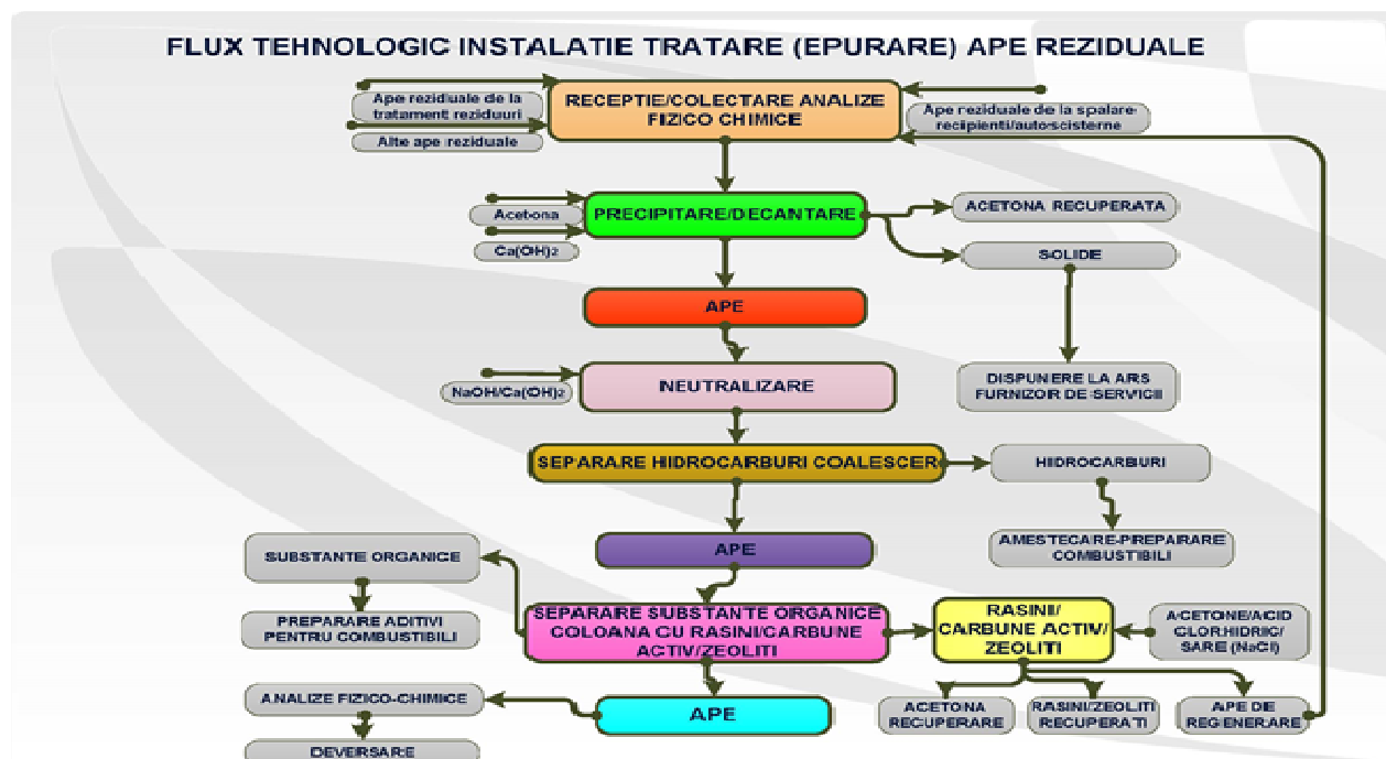
Figura 4: Instalatia de (tratare) epurare ape reziduale
