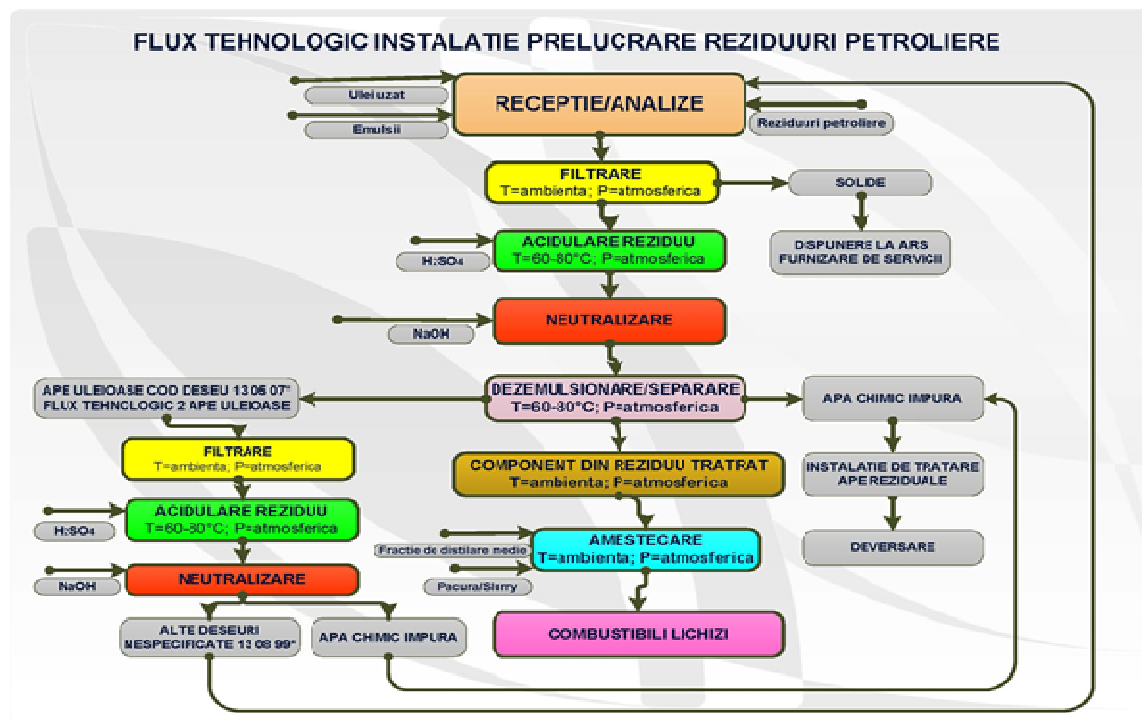
Figura 2: Flux tehnologic instalatie de prelucrare reziduuri
