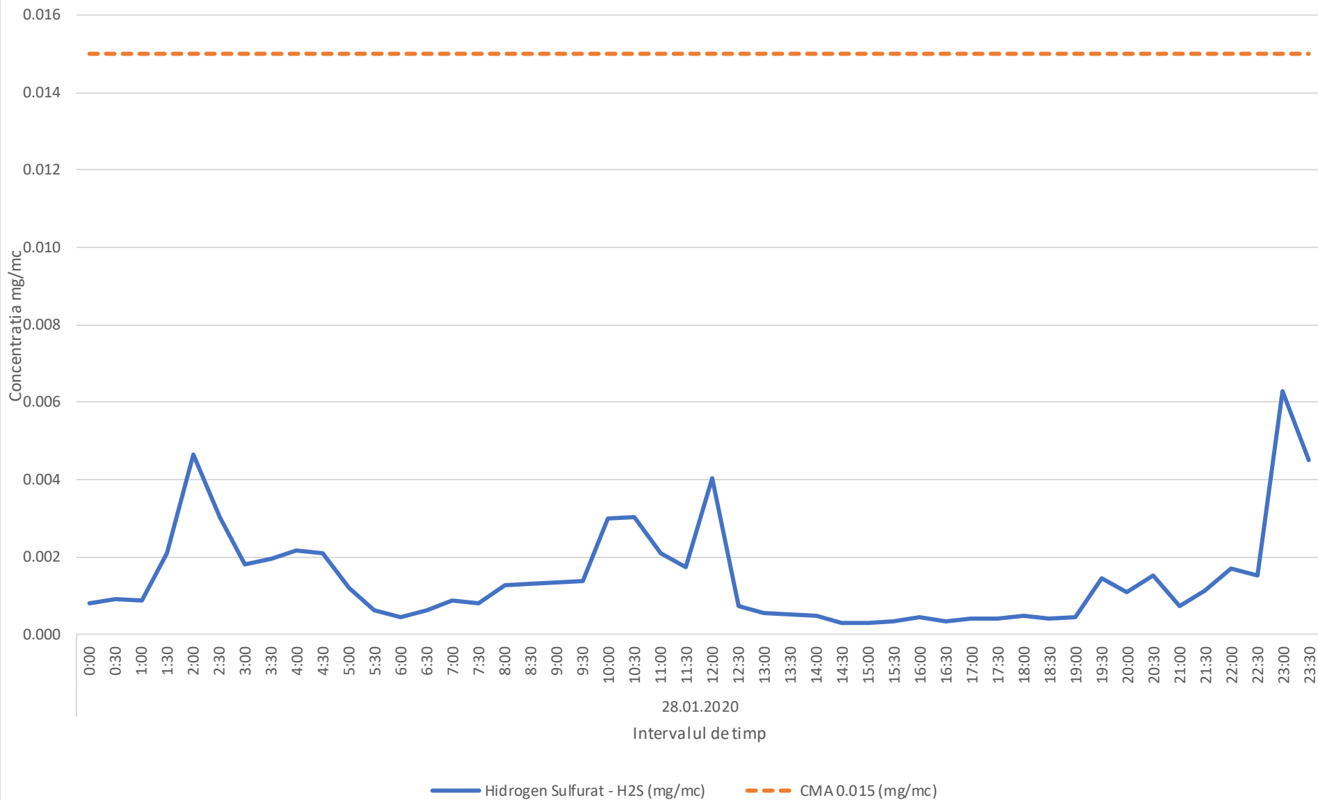
Variatia momentana (30 min.) a indicatorului H2S in data de 28.01.2020 - Comuna Barcanesti
