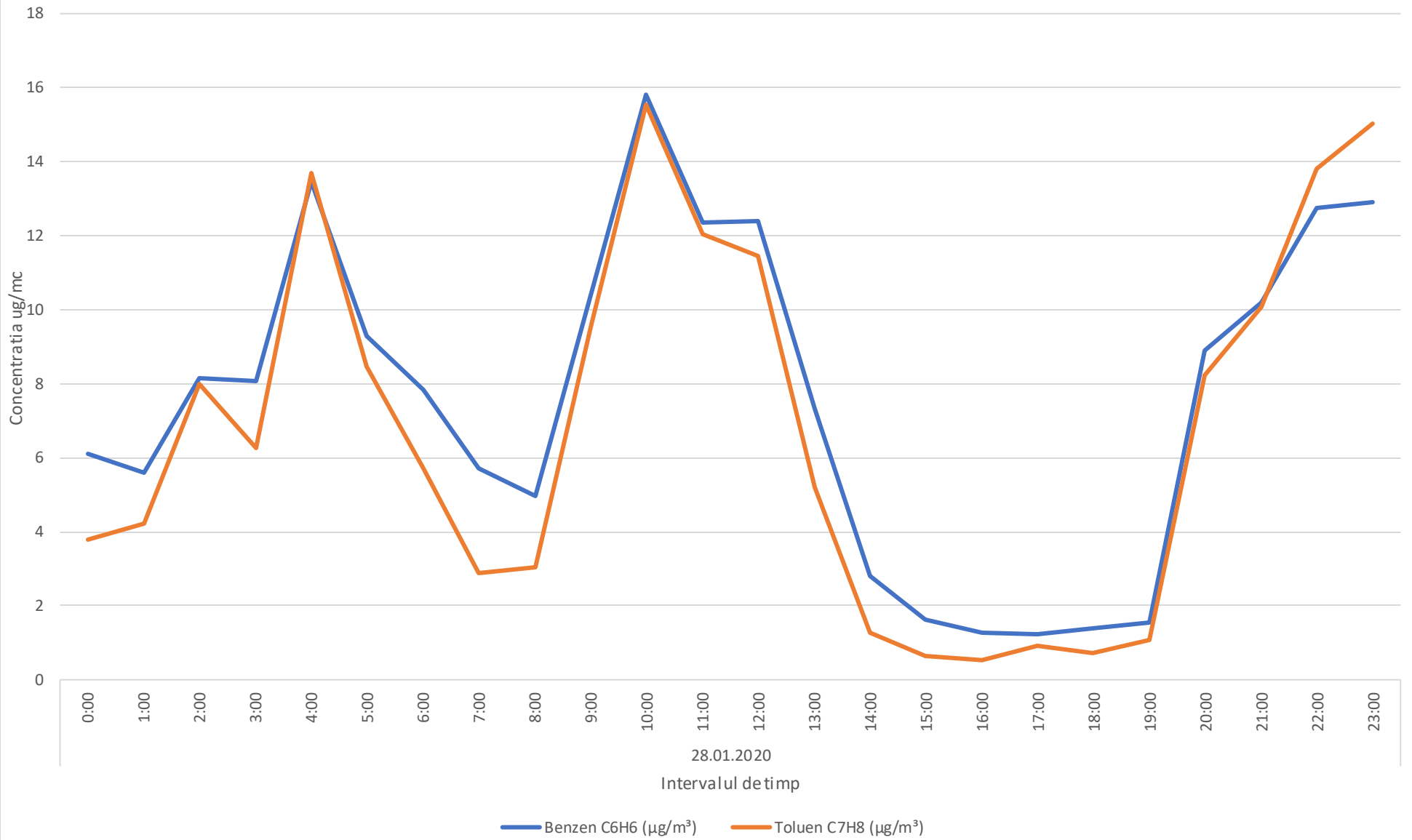
Variatia mediilor orare a indicatorilor C6H6,C7H8 in data de 28.01.2020 - Comuna Barcanesti
