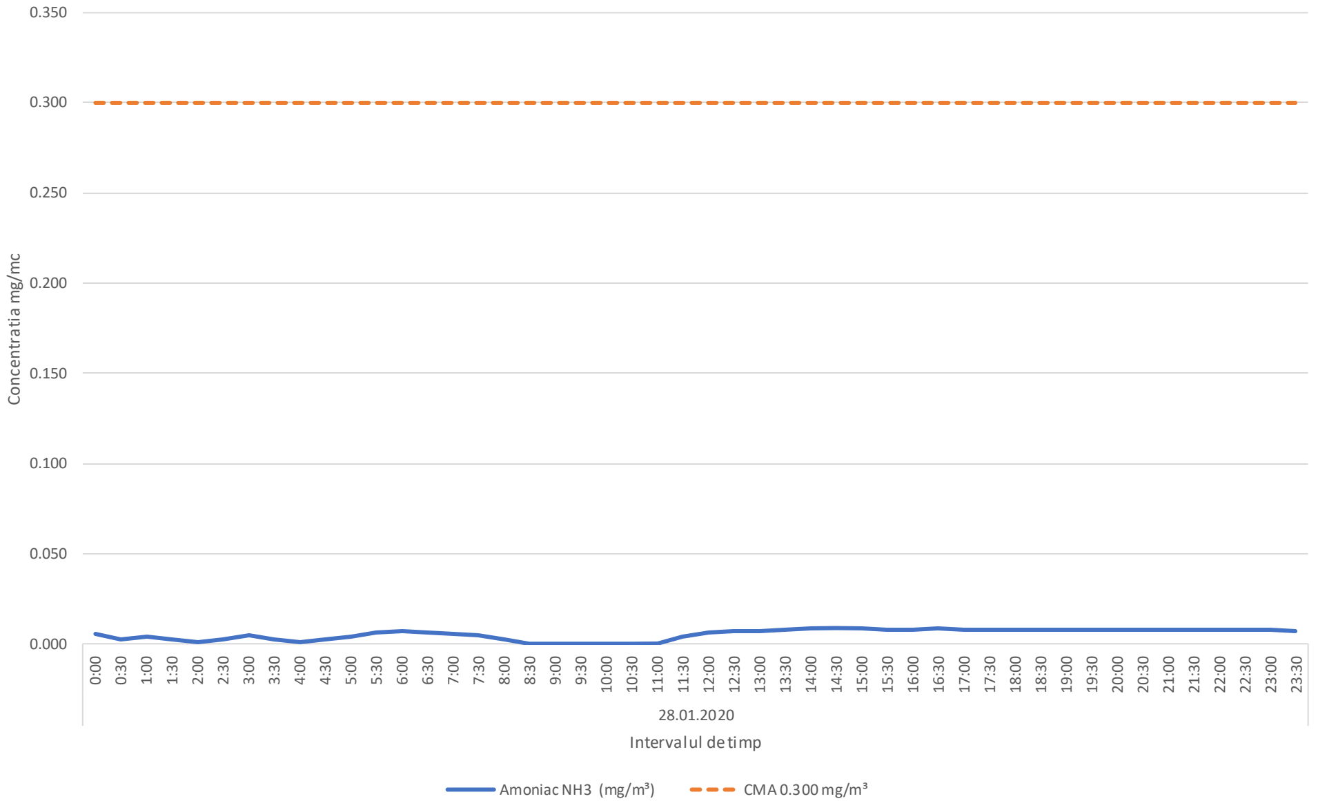
Variatia momentana (30 min.) a indicatorului NH3 in data de 28.01.2020 - Comuna Barcanesti
