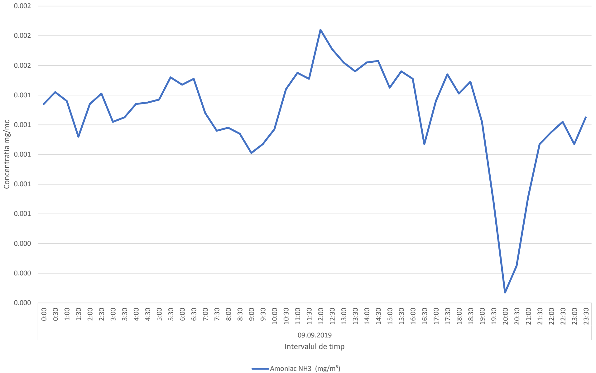
Variatia momentana (30 min.) a indicatorului NH3 in data de 09.09.2019- zona Comunei Paulesti
