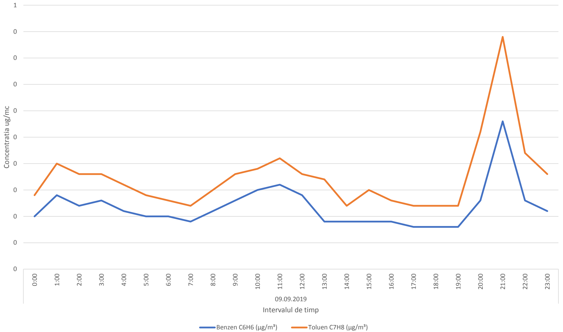
Variatia mediilor orare a indicatorilor C6H6,C7H8 in data de 09.09.2019- zona Comunei Paulesti
