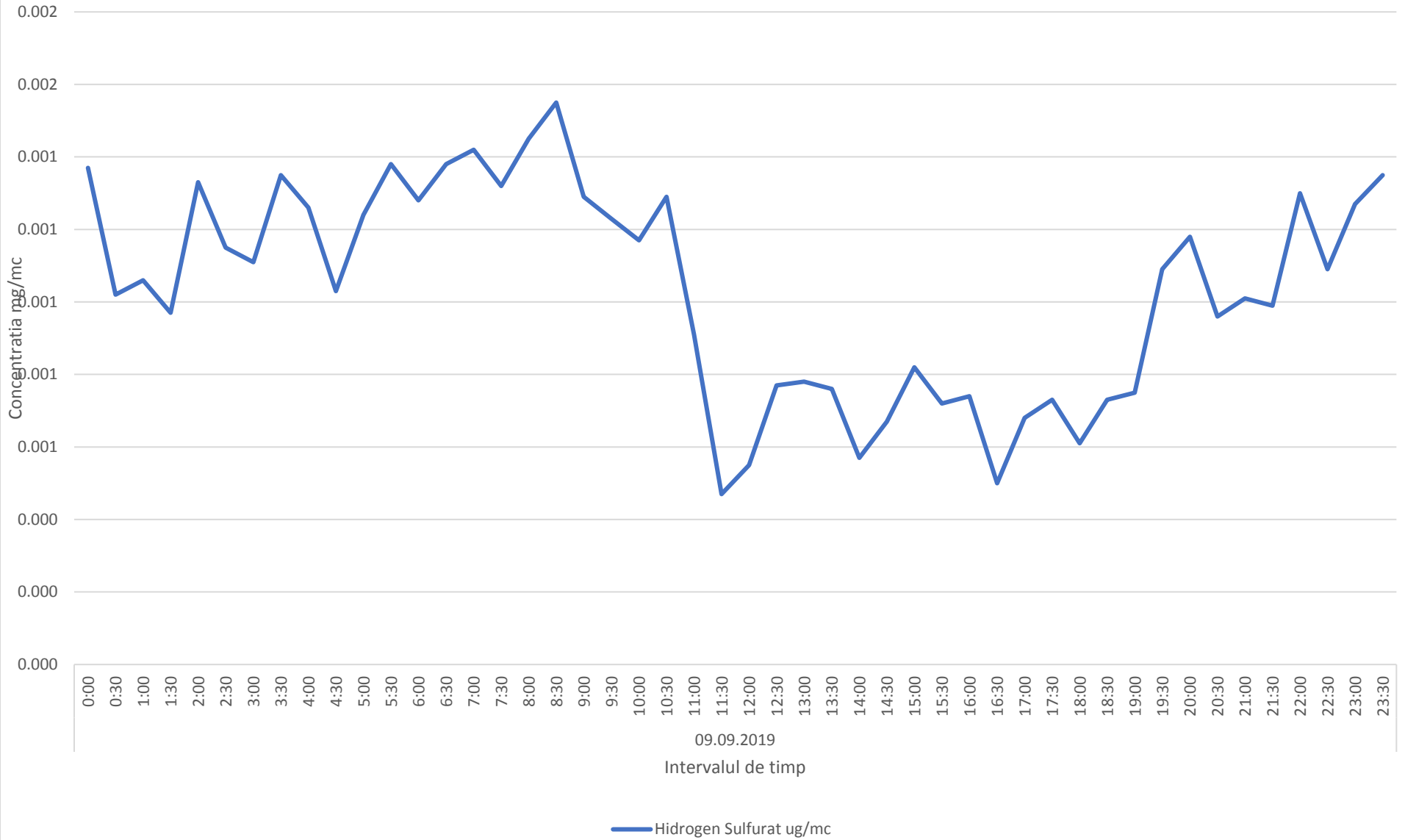
Variatia momentana (30 min.) a indicatorului H2S in data de 09.09.2019- zona Comunei Paulesti
