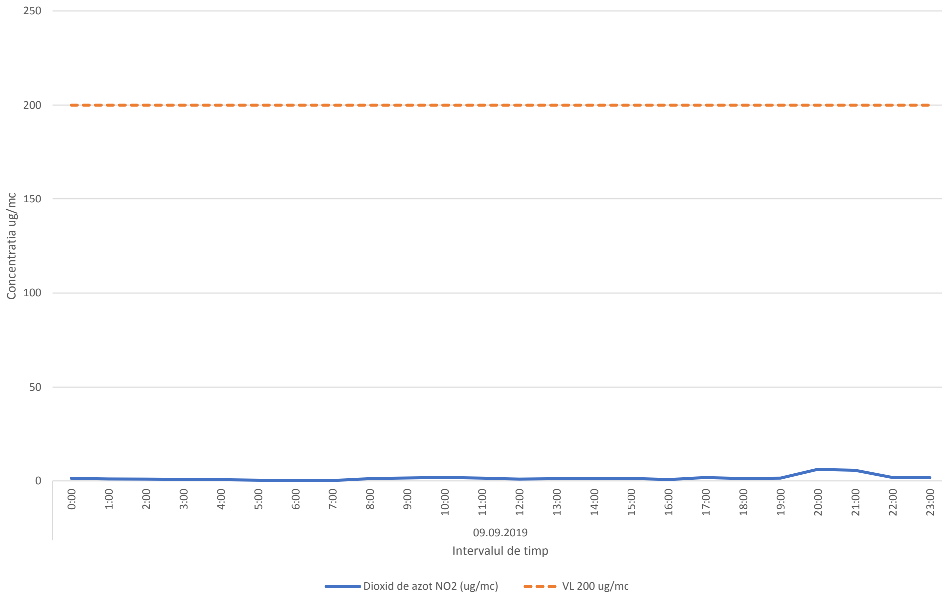
Variatia mediilor orare ale indicatorului NO2 in data de 09.09.2019- zona Comunei Paulesti
