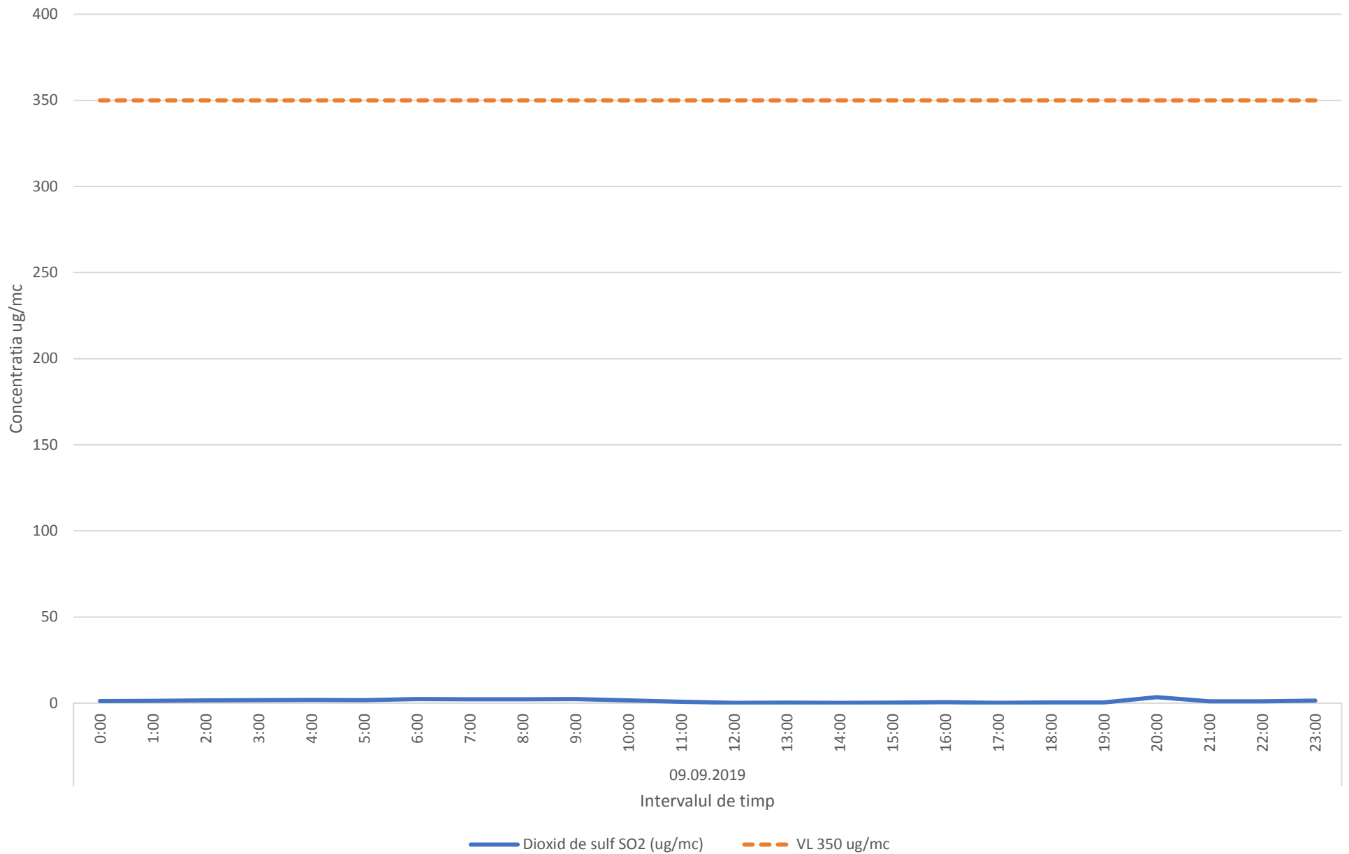
Variatia mediilor orare ale indicatorului SO2 in data de 09.09.2019- zona Comunei Paulesti
