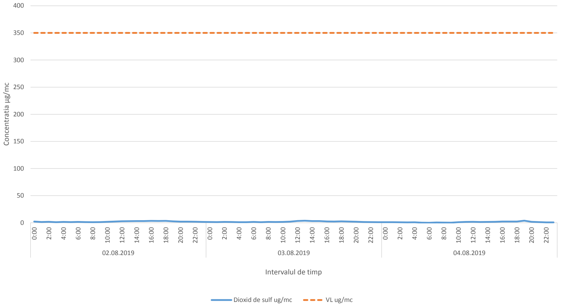
Variatia orara a indicatorului SO2 in perioada 02.08.2019-04.08.2019 - zona de nord a Municipiului Ploiesti
