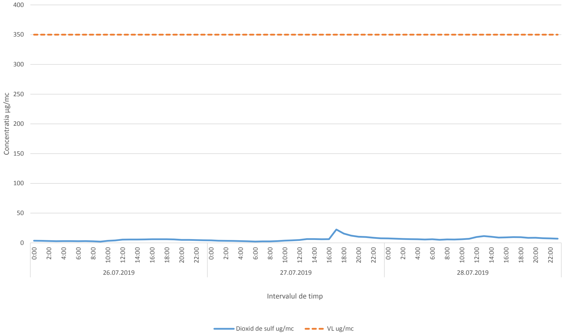
Variatia orara a indicatorului SO2 in perioada 26.07.2019-28.07.2019 - zona de nord a Municipiului Ploiesti
