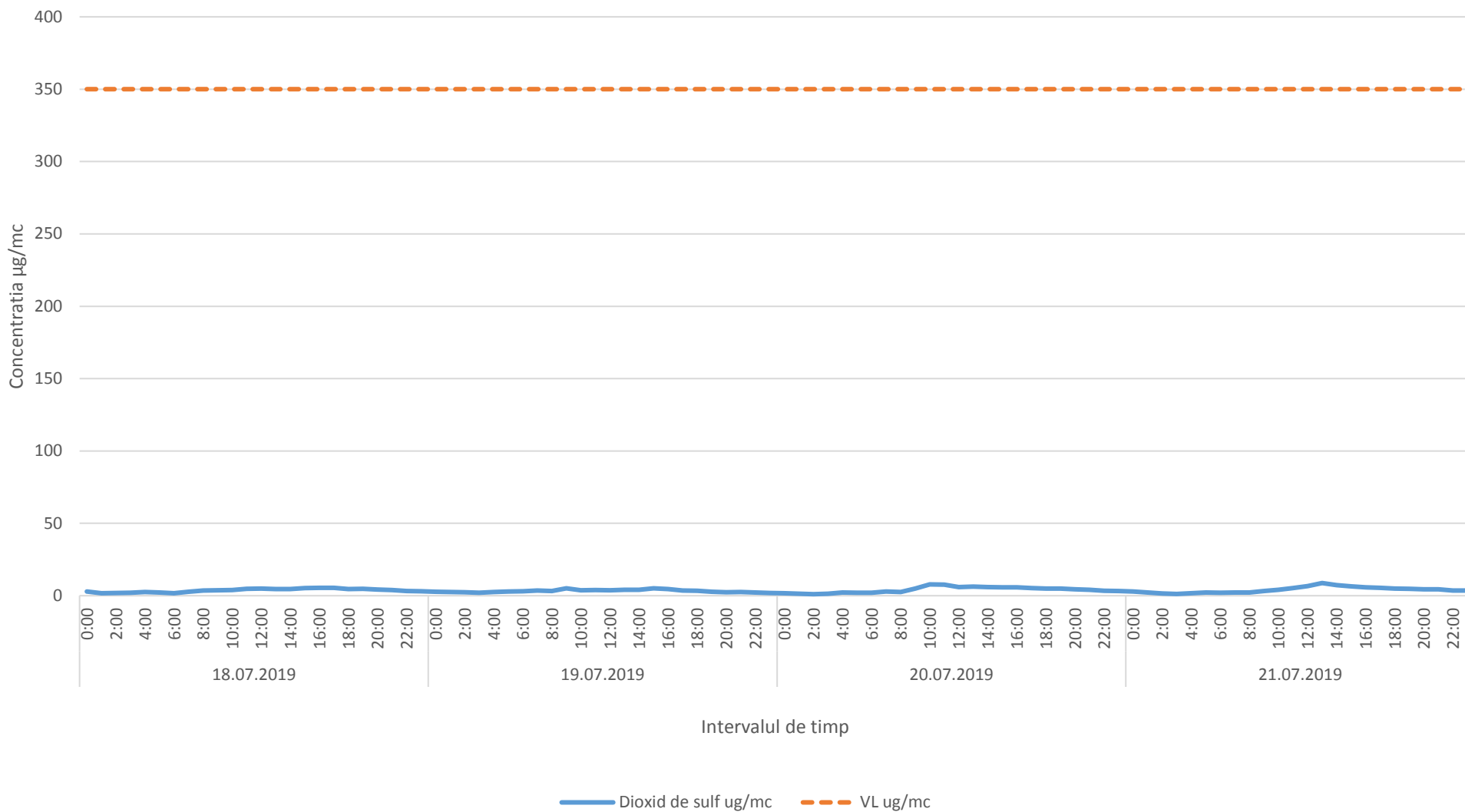
Variatia orara a indicatorului SO2 in perioada 18.07.2019-21.07.2019- zona de nord a platformei industriale Brazi
