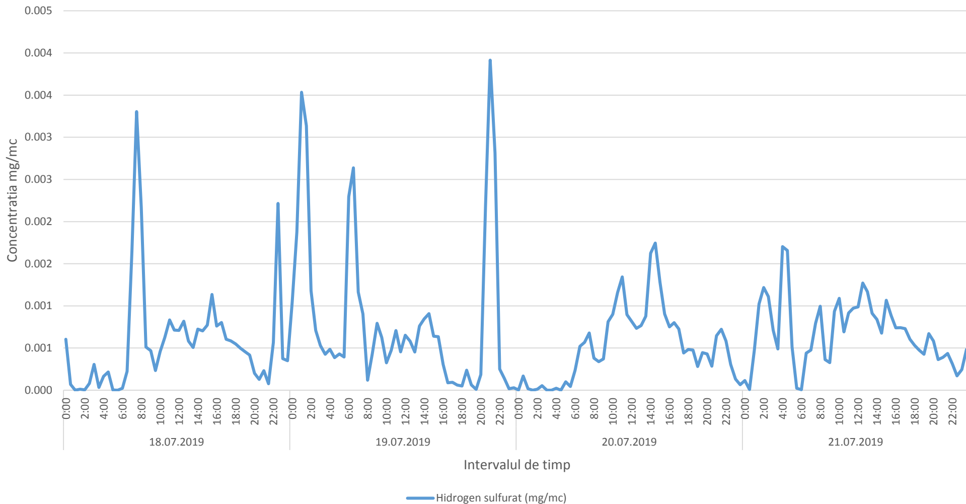
Variatia momentana (30 min.) a indicatorului H2S in perioada 18.07.2019-21.07.2019- zona de nord a platformei industriale Brazi
