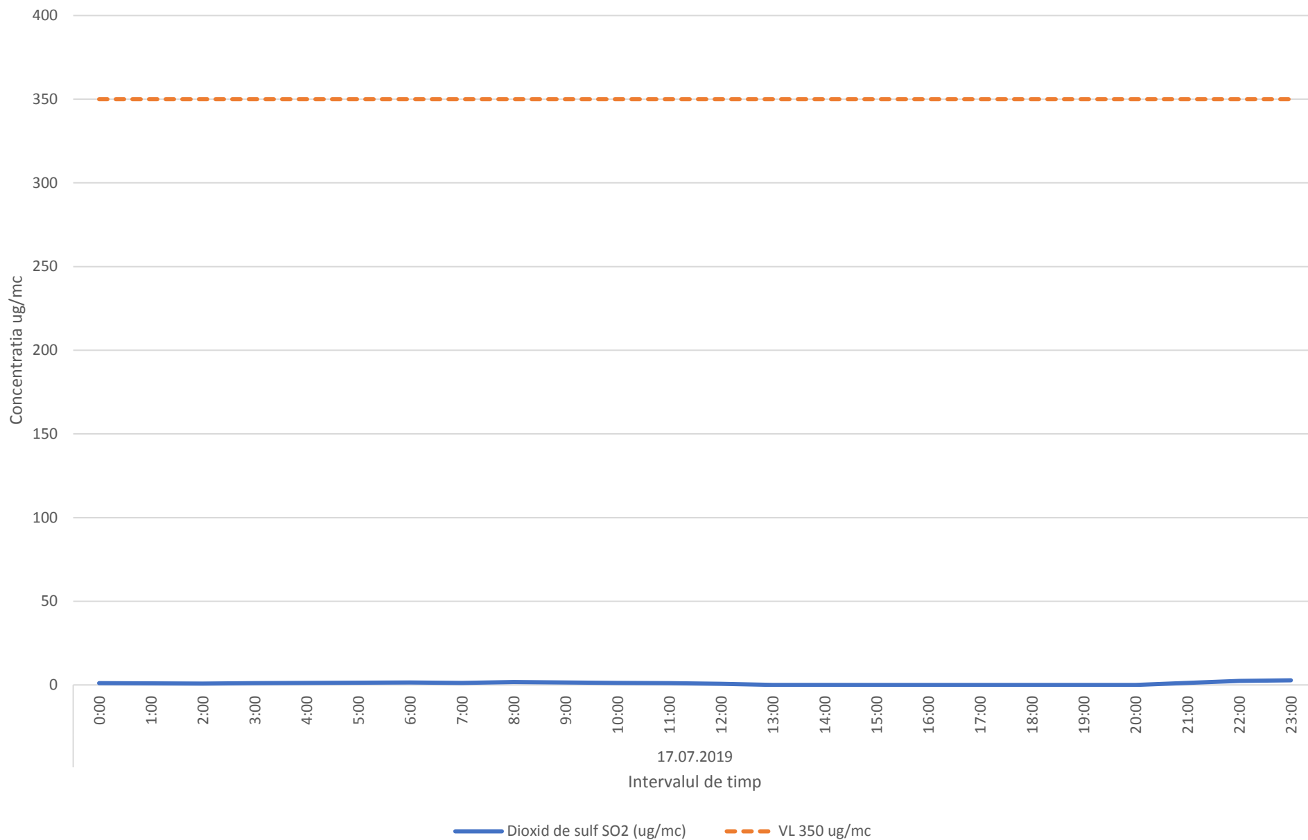
Variatia medilor orare ale indicatorului SO2 in data de 17.07.2019 - zona de nord-vest a platformei industriale Brazi
