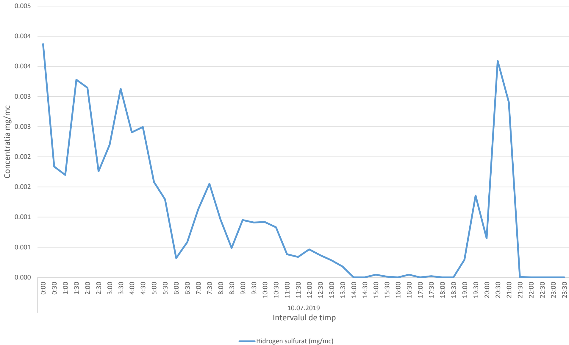
Variatia momentana (30 min.) a indicatorului H2S in data de 10.07.2019 - zona de nora a platformei industriale Brazi
