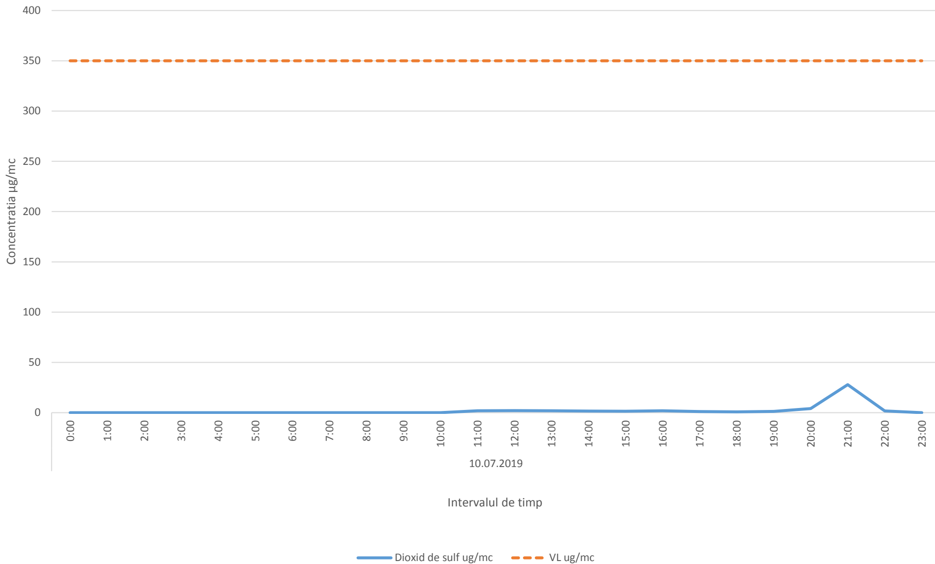
Variatia orara a indicatorului SO2 in data de 10.07.2019 - zona de nora a platformei industriale Brazi
