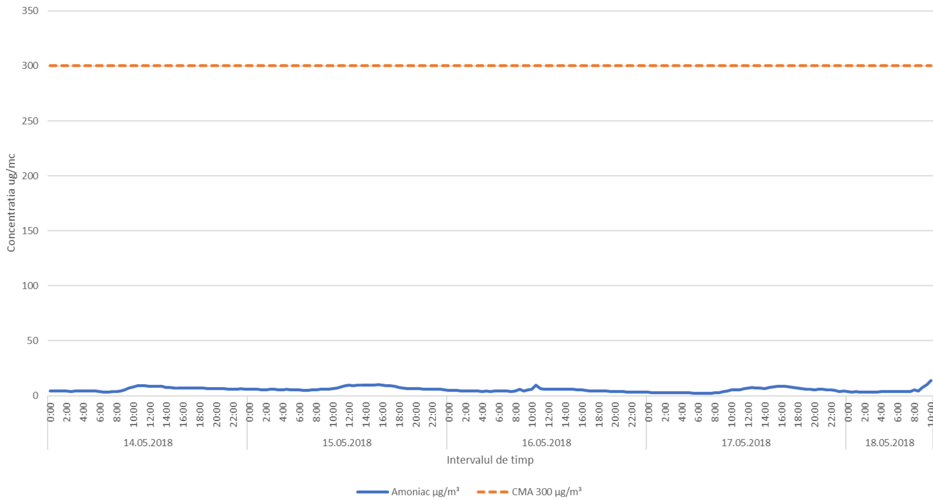
Variatia indicatorului NH3 in intervalul 14.05.2018 - 18.05.2018 in zona cartierului Mihai Bravu
