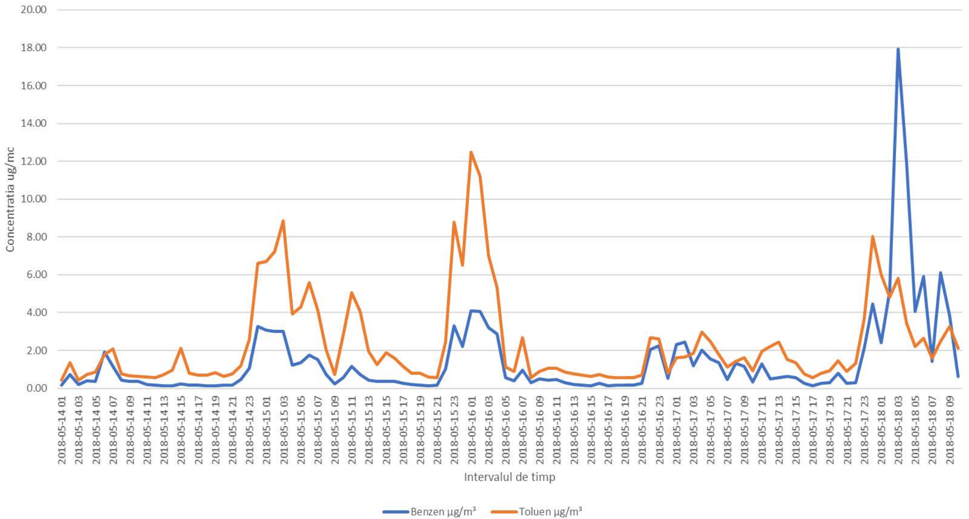
Variatia indicatorilor Benzen/Toluen in in intervalul 13.05.2018 - 18.05.2018 in zona cartierului Mihai Bravu
