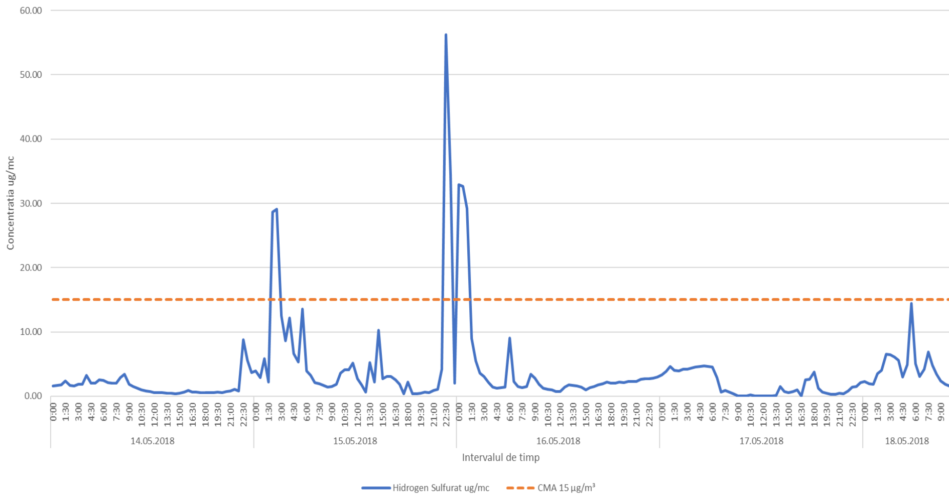
Variatia indicatorului H2S in intervalul 14.05.2018 - 18.05.2018 in zona cartierului Mihai Bravu
