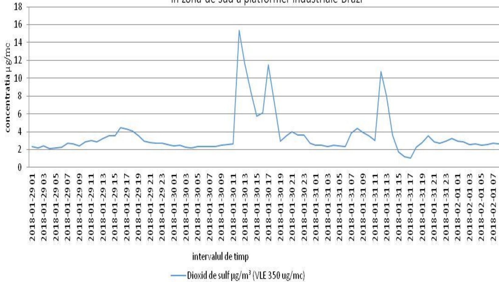
Variatia indicatorului dioxid de sulf in perioada 29.02.2018-04.02.2018 in zona de sud a platformei industriale Brazi
