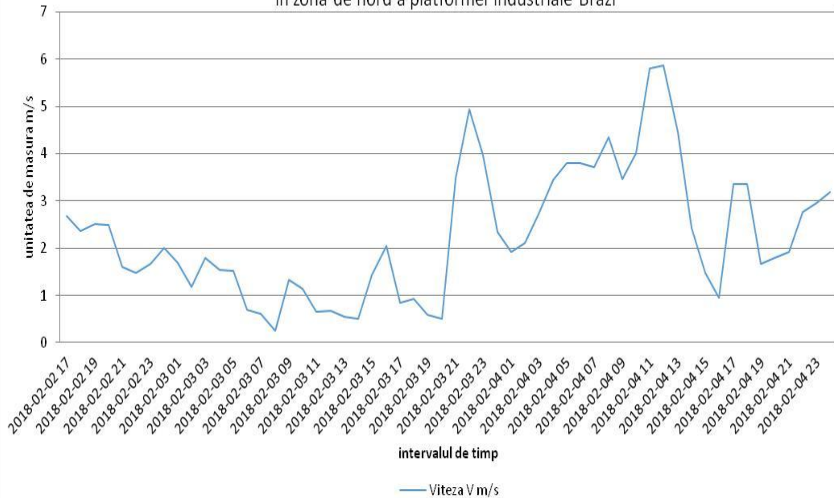
Variatia vitezei vantului in perioada 02.02.2018-04.02.2018 in zona de nord a platformei industriale Brazi
