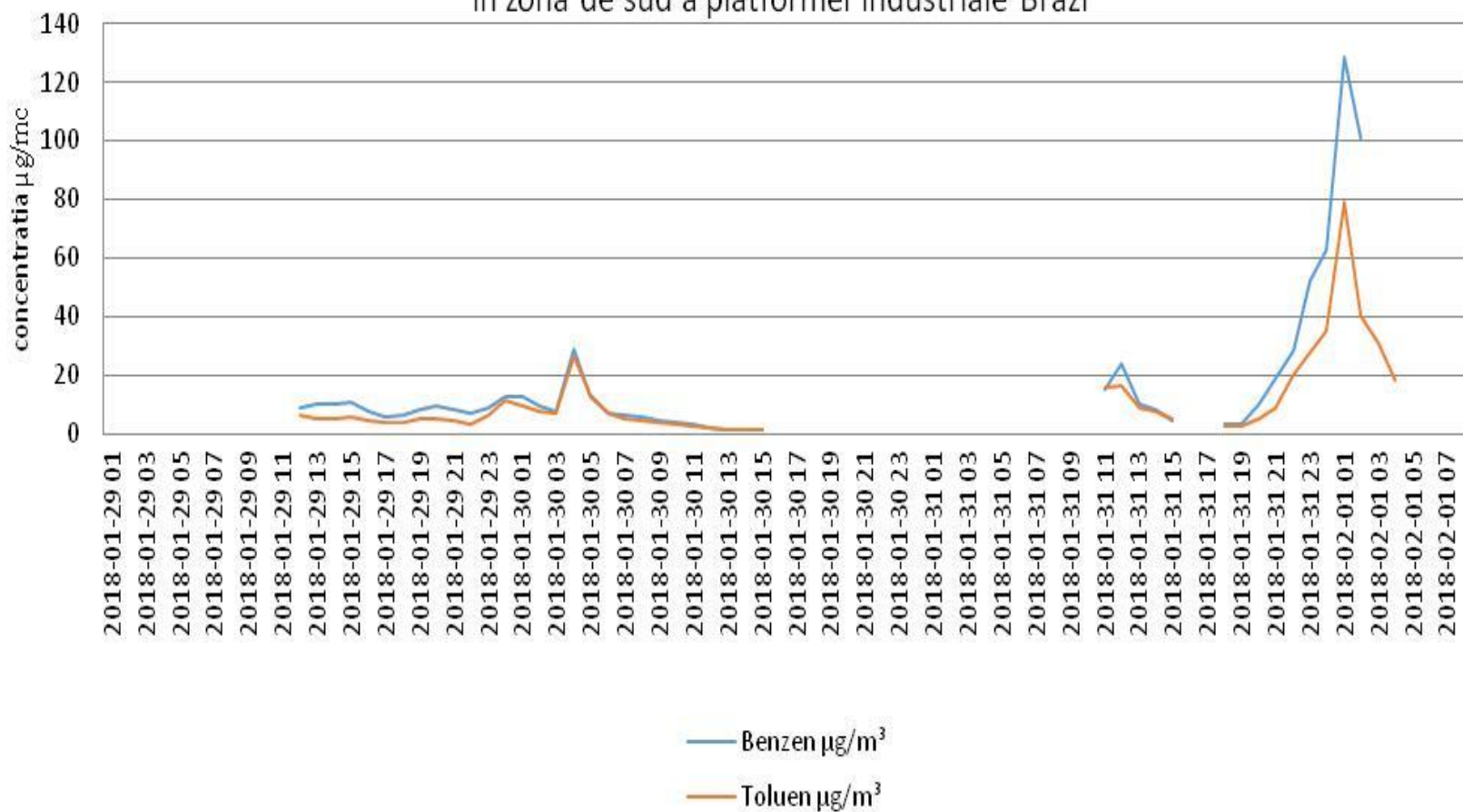
Variatia indicatorilor benzen si toluen in perioada 29.01.2018-02.02.2018 in zona de sud a platformei industriale Brazi
