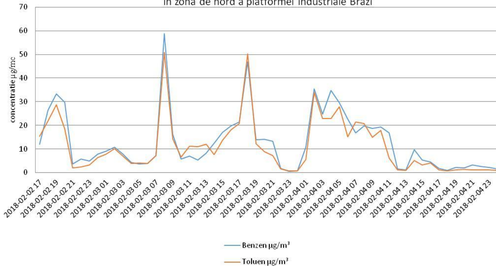
Variatia indicatorilor benzen si toluen in perioada 02.02.2018-04.02.2018 in zona de nord a platformei industriale Brazi
