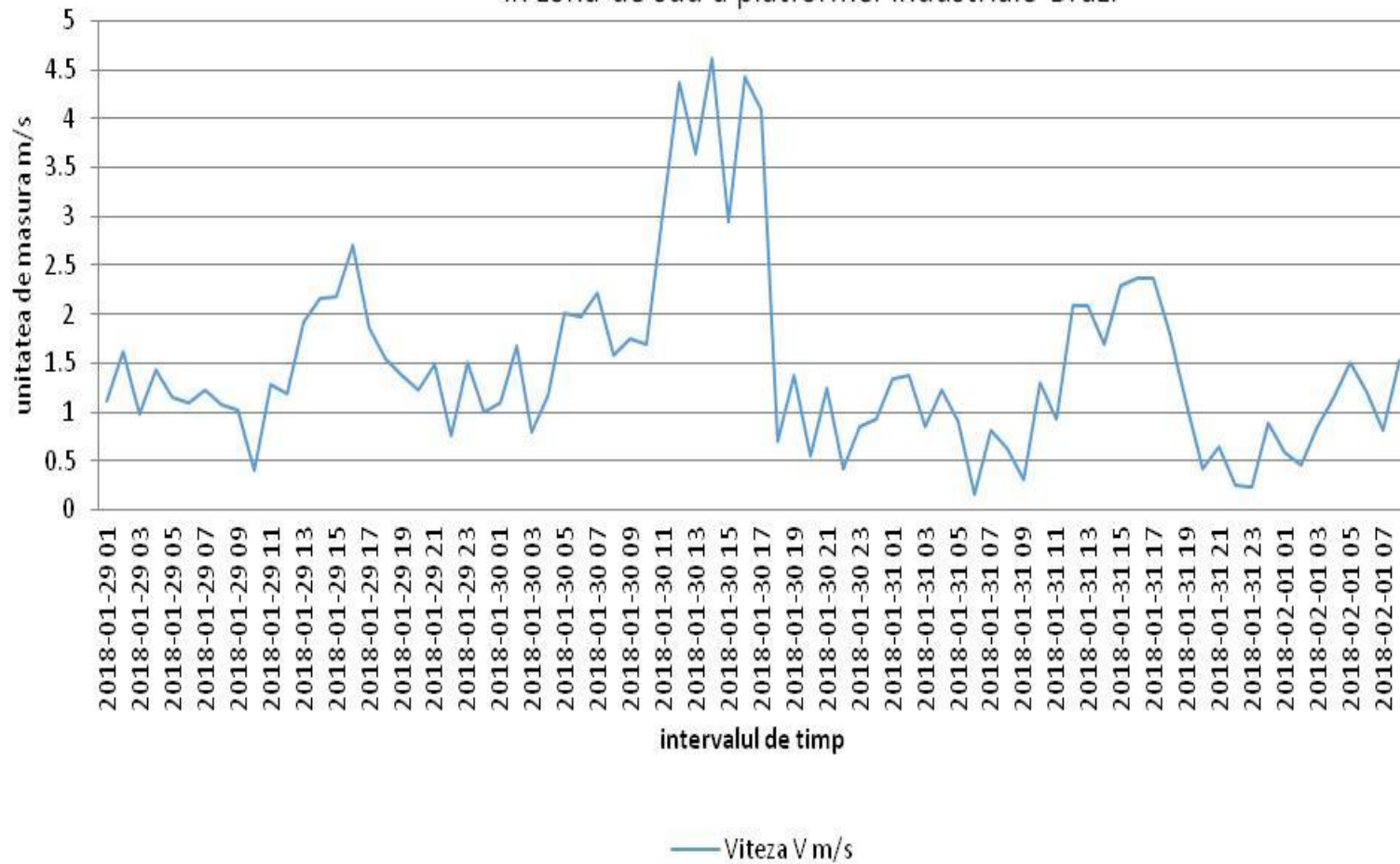
Variatia vitezei vantului in perioada 29.01.2018-02.02.2018 in zona de sud a platformei industriale Brazi
