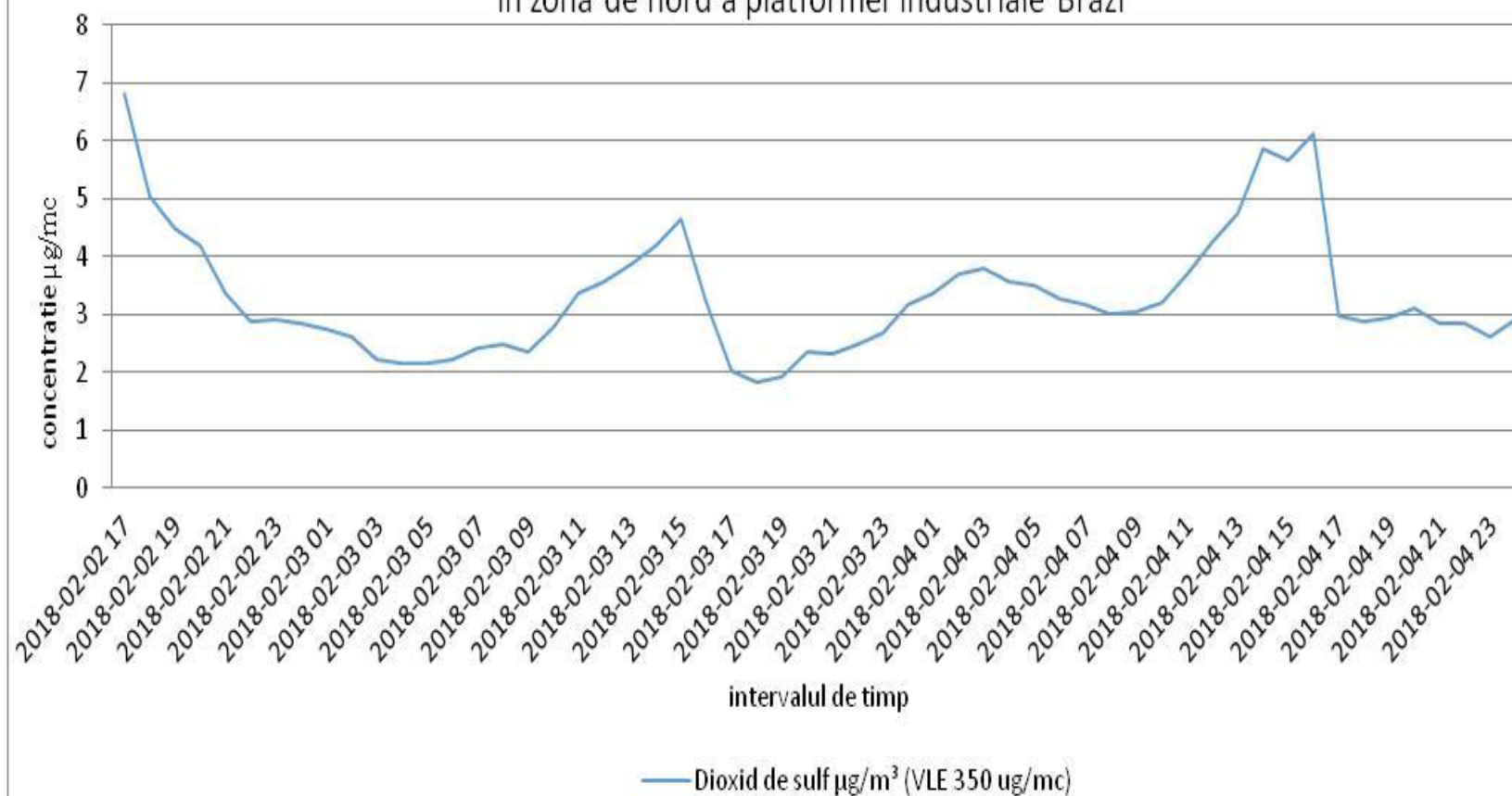
Variatia indicatorului dioxid de sulf in perioada 02.02.2018-04.02.2018 in zona de nord a platformei industriale Brazi
