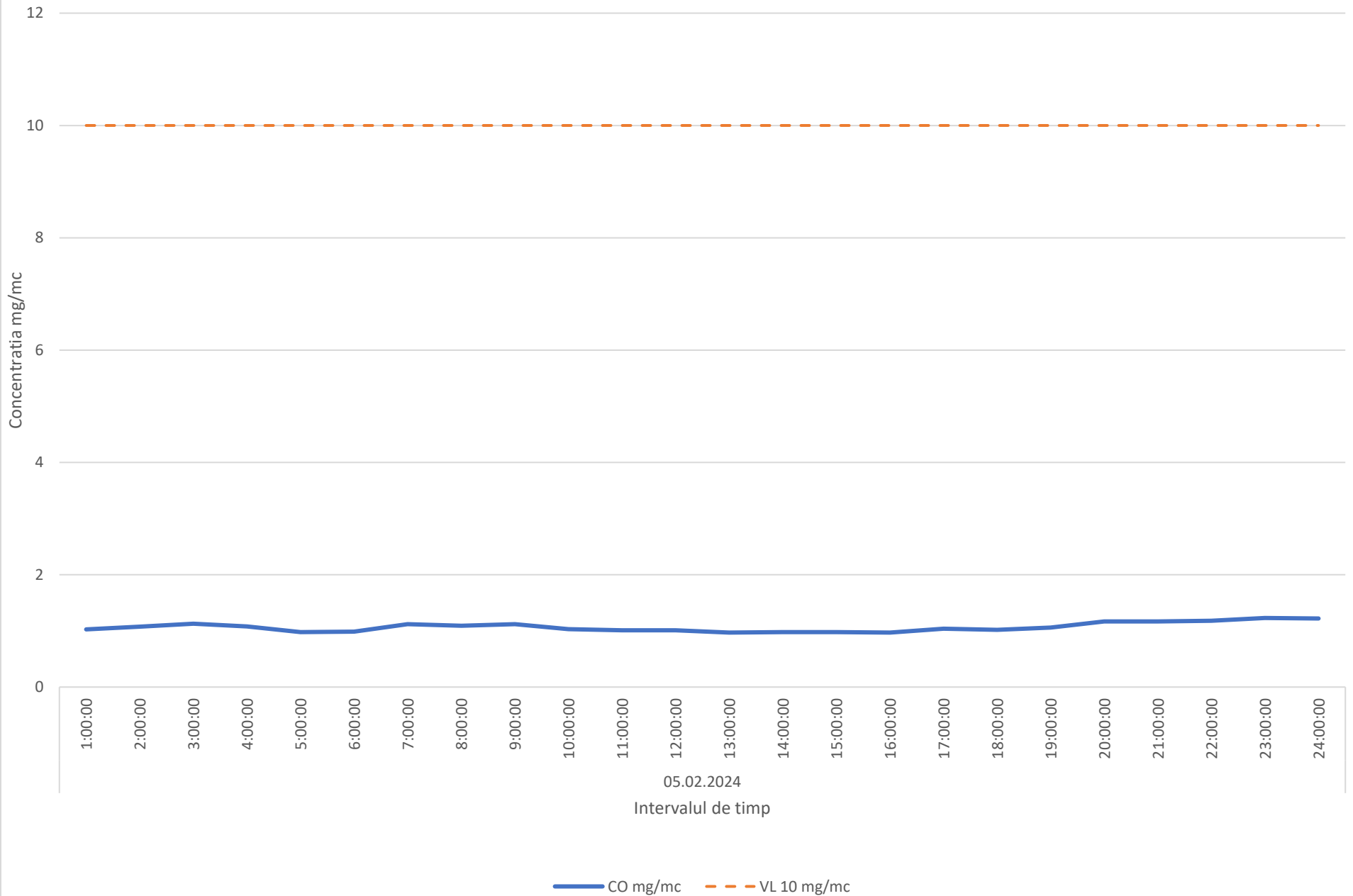
Variatia mediilor orare ale indicatorului CO in data de 05.02.2024 - Parcul Central, Municipiul Ploiesti
