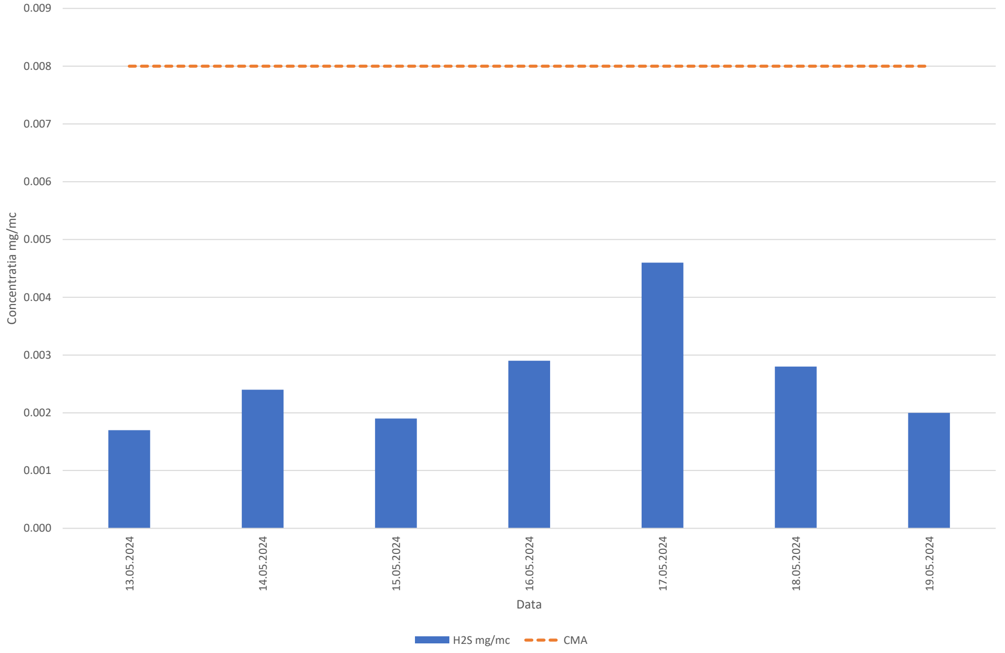
Variatia concentratiilor mediilor zilnice ale indicatorului H2S in perioada 13.05.2024-19.05.2024 - Str. Persani, Municipiul Ploiesti
