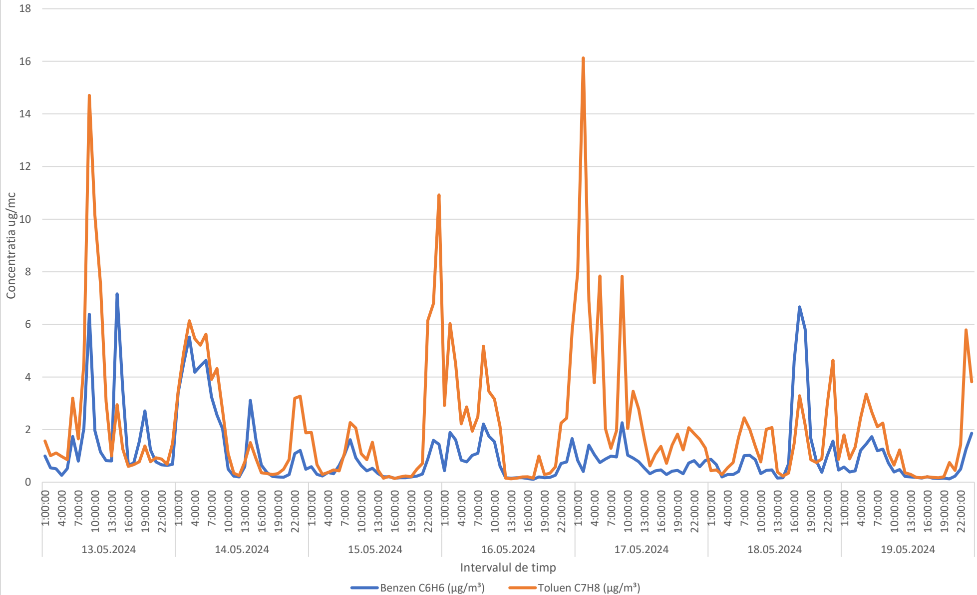
Variatia concentratiilor mediilor orare ale indicatorilor C6H6,C7H8 in perioada 13.05.2024-19.05.2024 - Str. Persani, Municipiul Ploiesti
